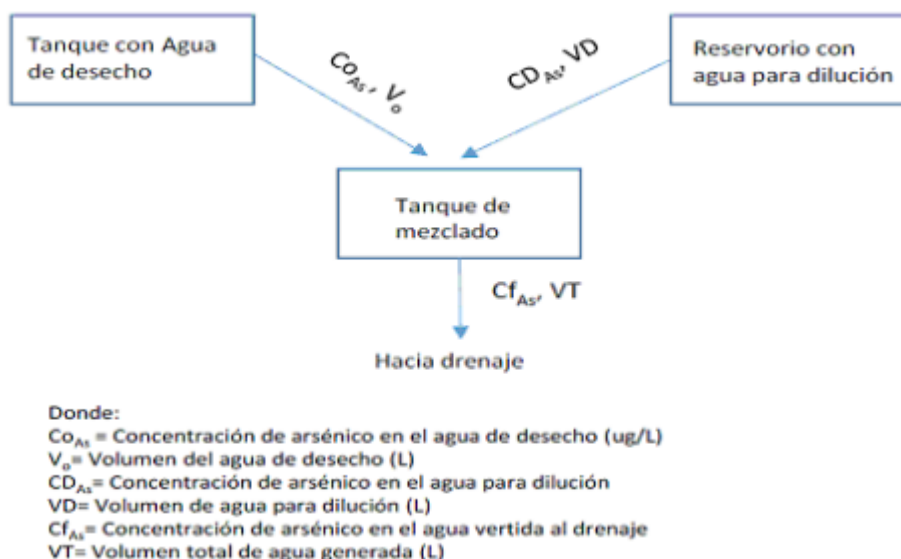
Figura G.3 Diagrama del balance de masa para la disolución de arsénico en el agua vertida a la red
